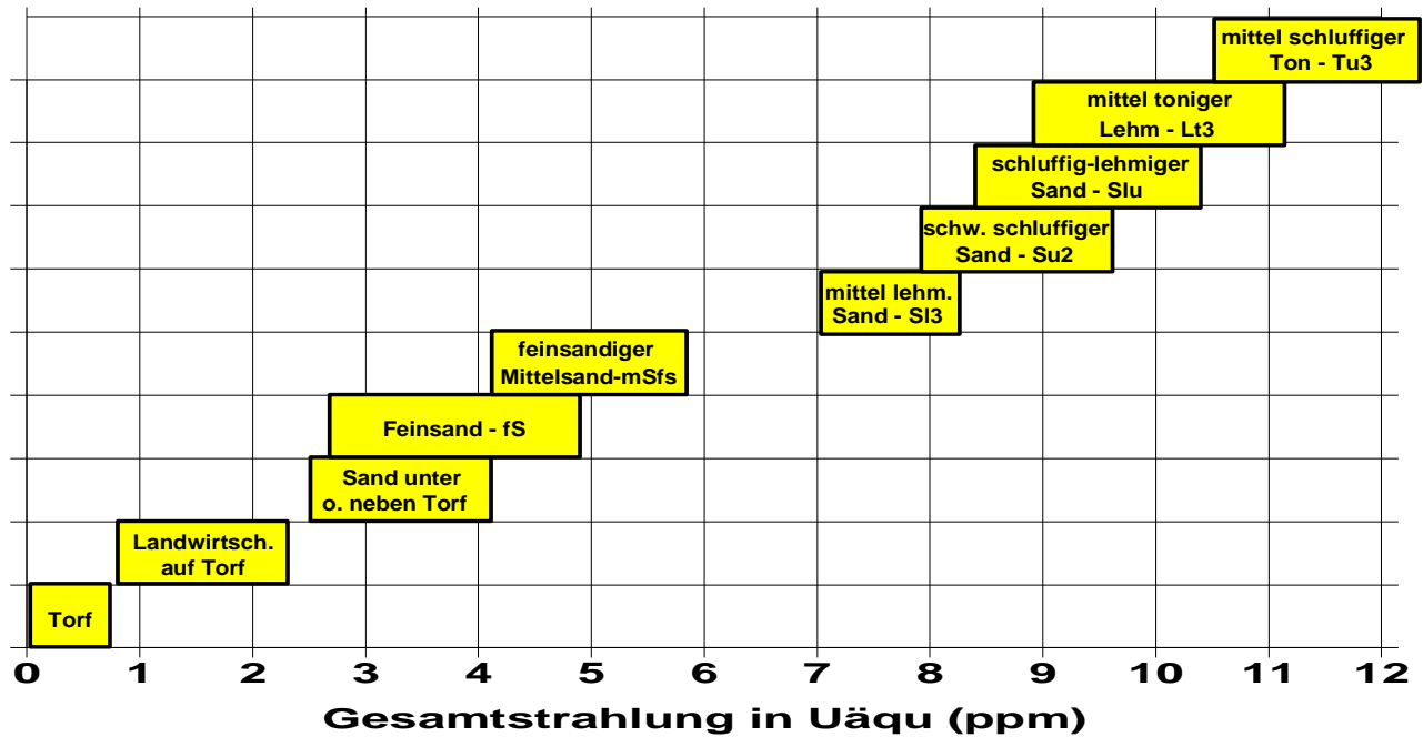
Abb. 8: Wertebereich der natürlichen \gamma -Aktivität von anstehenden Bodenarten
